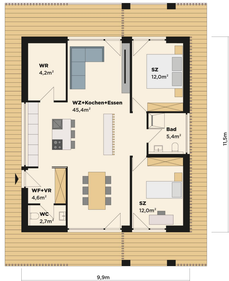
Grundriss
